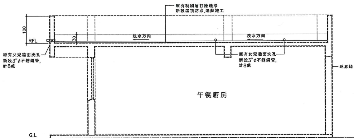
A 剖面圖 S:1/40
