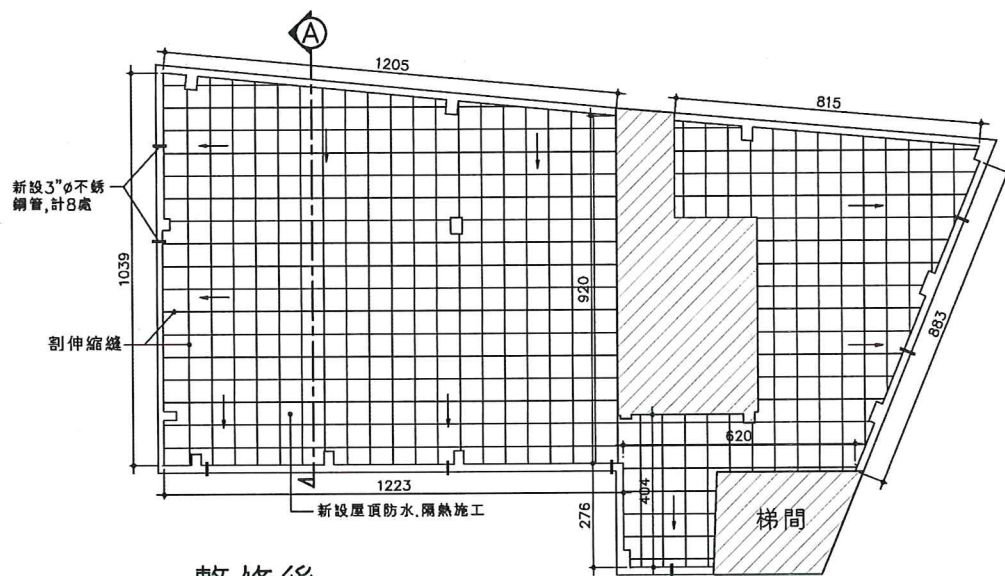
整修後 午餐廚房屋頂平面圖 S:1/100
